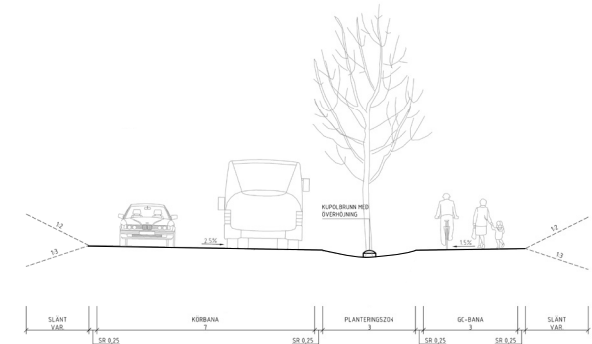
Principsektion Kolonnvägen.
