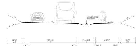
Principsektion ny lokalgata.
