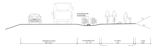
Principsektion Kungsbäcksvägen.
