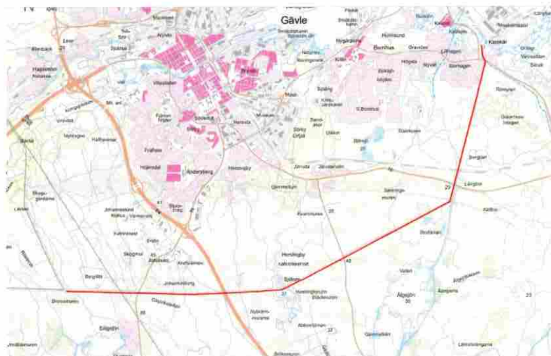
Karta som visar den aktuella sträckningen för nätkoncessionen från Nätstämur i väster till Karskär i öster.
